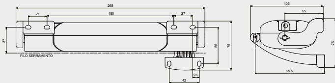
Fenêtre à soufflet: Dimensions et trous de fixation
