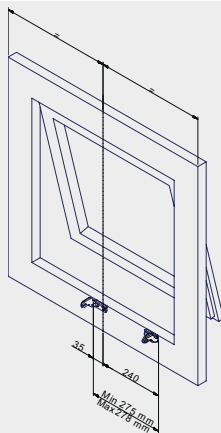
Fenêtre à l'italienne:
